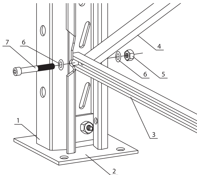
Рис 3. Установка раскосов.
